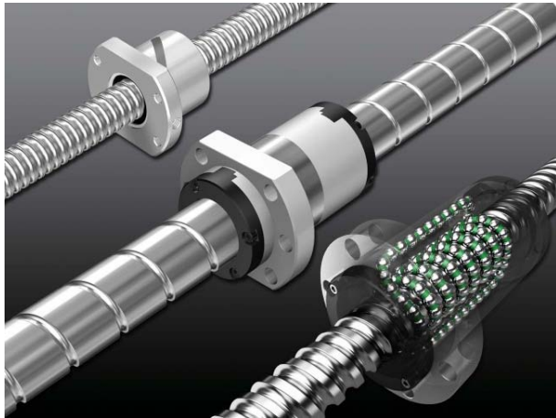
Ball Screw ボールねじ
