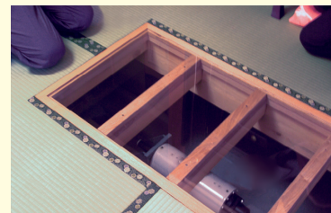
自宅にも免震装置を設置。お客様にご覧いただけるよう、畳の一部をガラス張りに。
