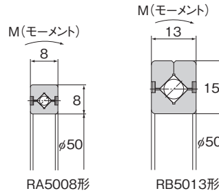
クロスローラーリング
