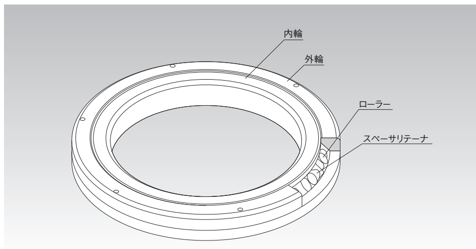
図1 クロスローラーリングRB形の構造
