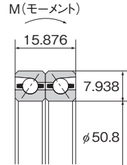
アンギュラ玉軸受
