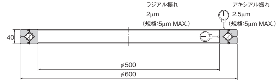
RB50040CCO USP形の内輪回転精度
