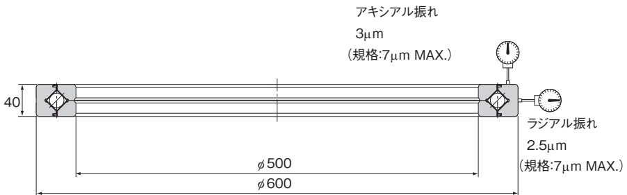
RE50040CCO USP形の外輪回転精度
