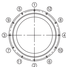
図1 締付順序
